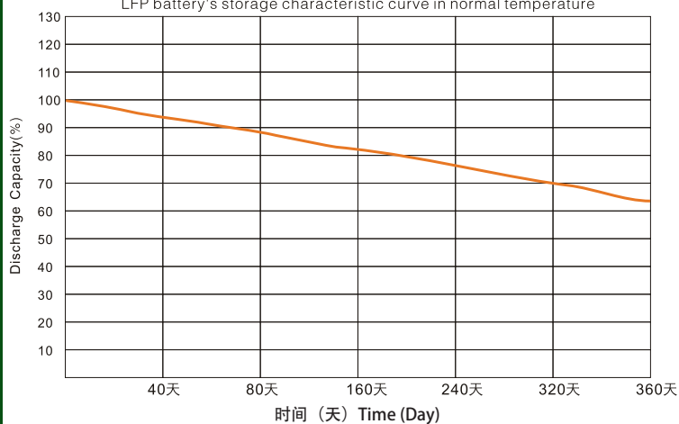
在常温环境下 LFP类电池的存储特性曲线
