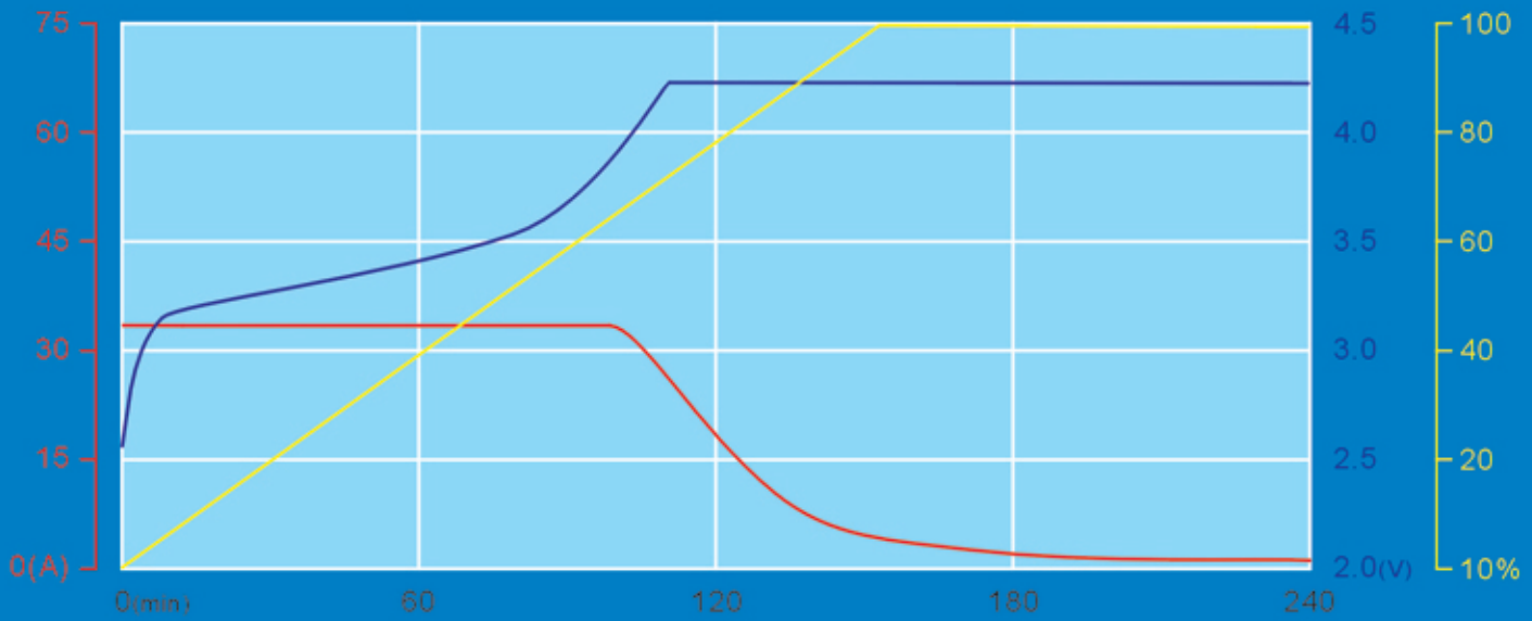
TS-LFP60AHA在25°C環境下的充電特性 TS-LFP60AHA CHARGE AT TEMPERATURE OF 25°C
