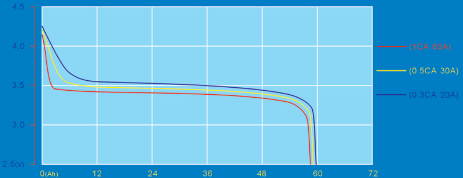
TS-LFP60AHA在25°C環境下的放電特性 TS-LFP60AHA DISCHARGE AT TEMPERATURE OF 25°C
